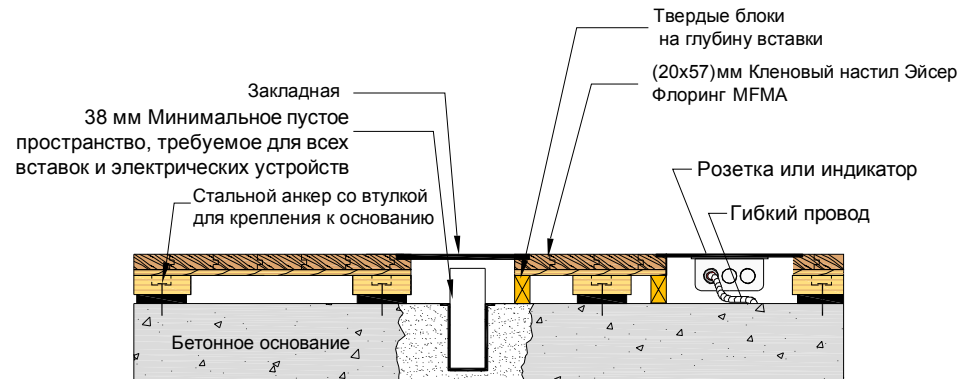
Установка оборудования
